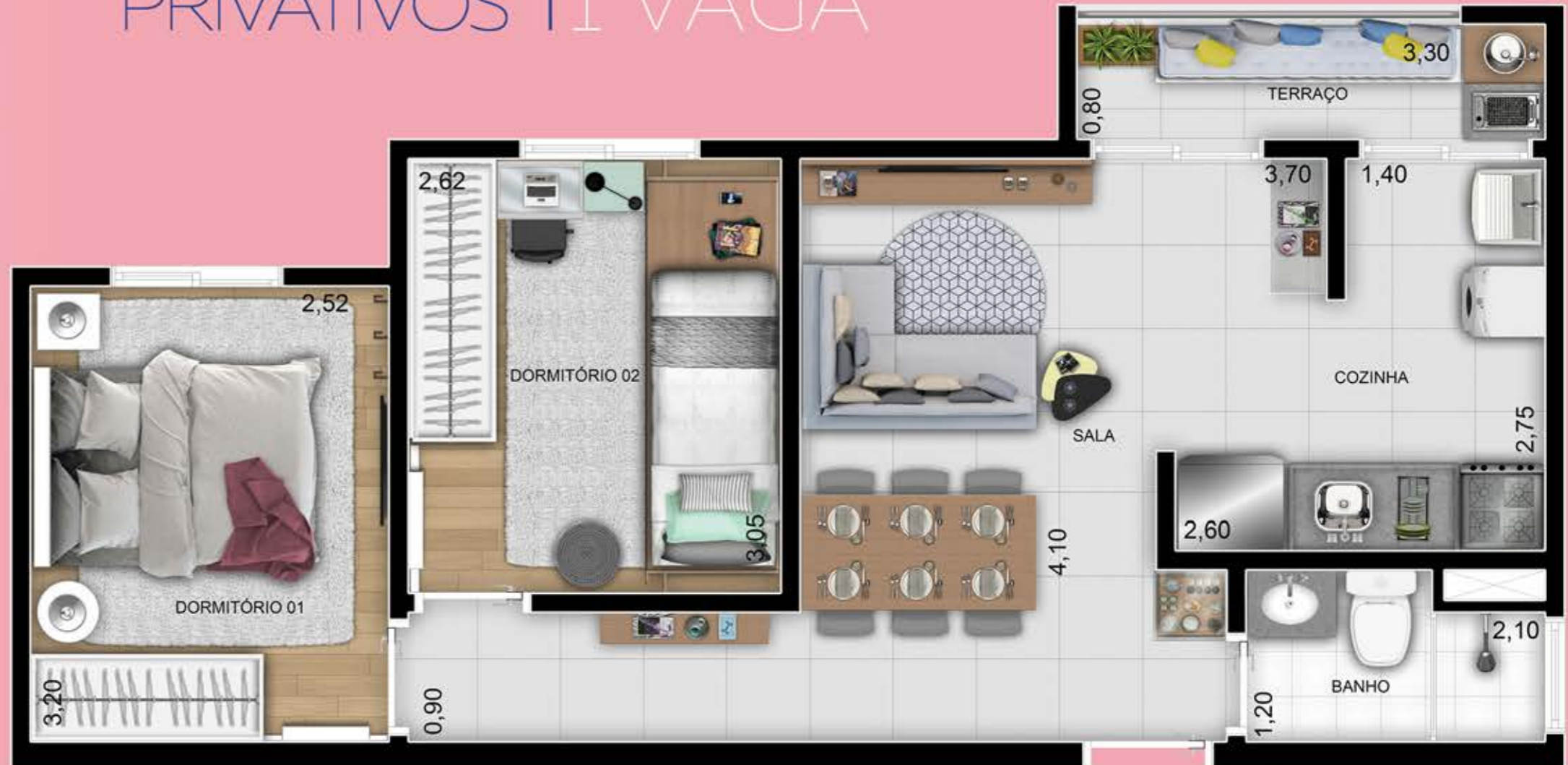
Ilustração da planta tipo. Móveis, objetos de decoração e utensílios, são meramente ilustrativos e não integram o memorial descritivo. Medidas de face a face em metros.
